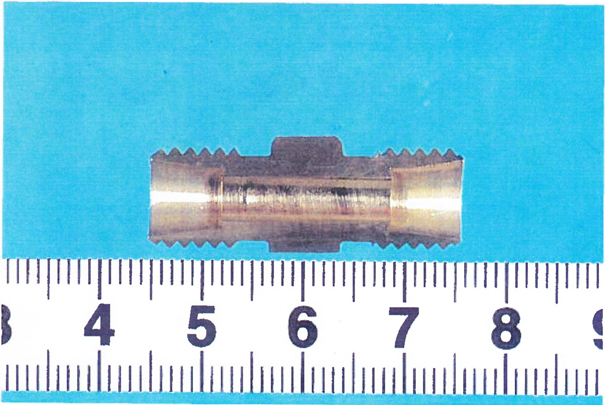
写真 2-3 1000ppm 浸漬後の真鍮
